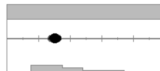
Erkennung einer Aluminium-Aufreiβblase (ID 30)
